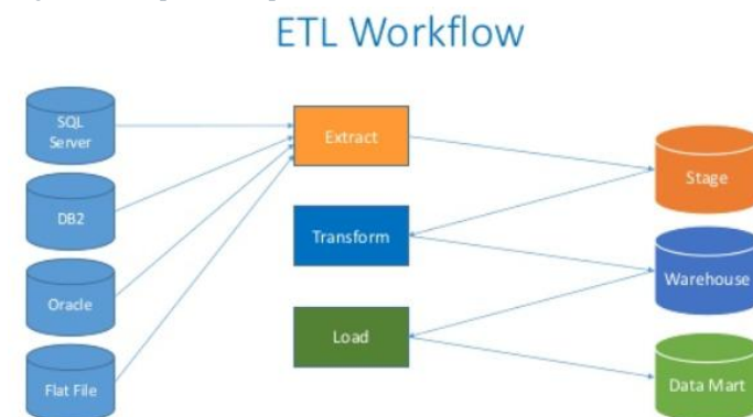
Figura 20: Esquema del proceso ETL básico.
