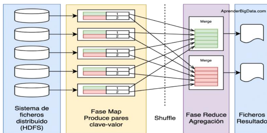
Figura 29: Funcionamiento de MapReduce
