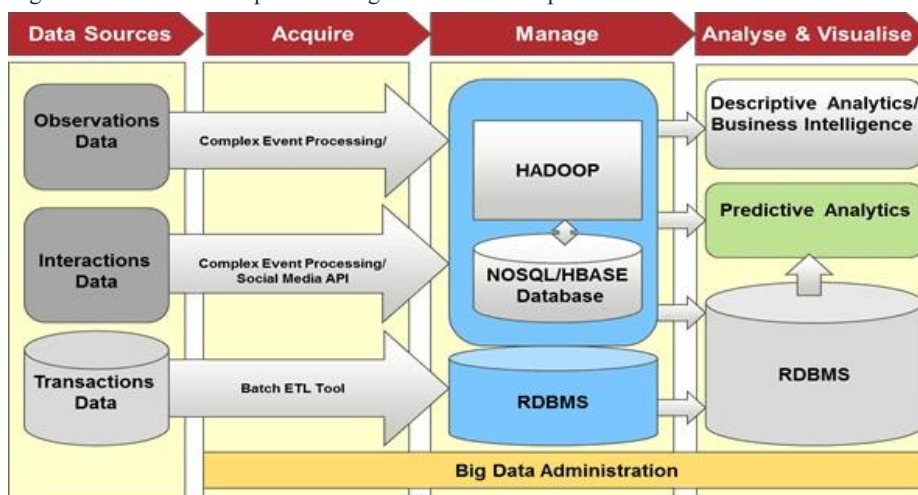
Figura 22: Variante de arquitectura big data de cuatro capas
