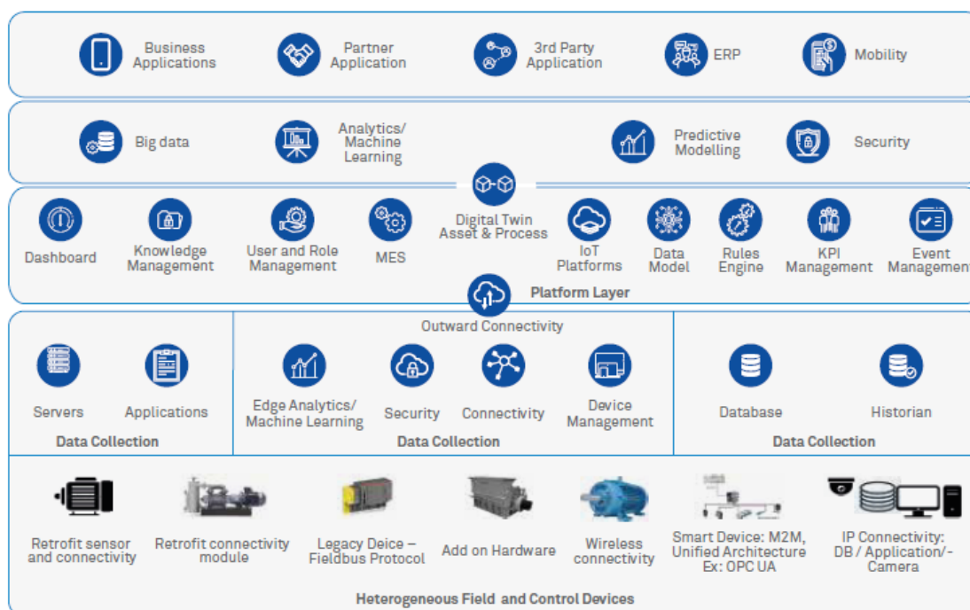
Figura 23: Ejemplo de arquitectura IoT industrial
