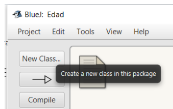
Figura 1.12 Nueva Clase
