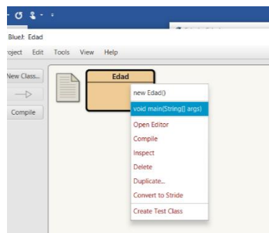
Figura 1.15 Método main
