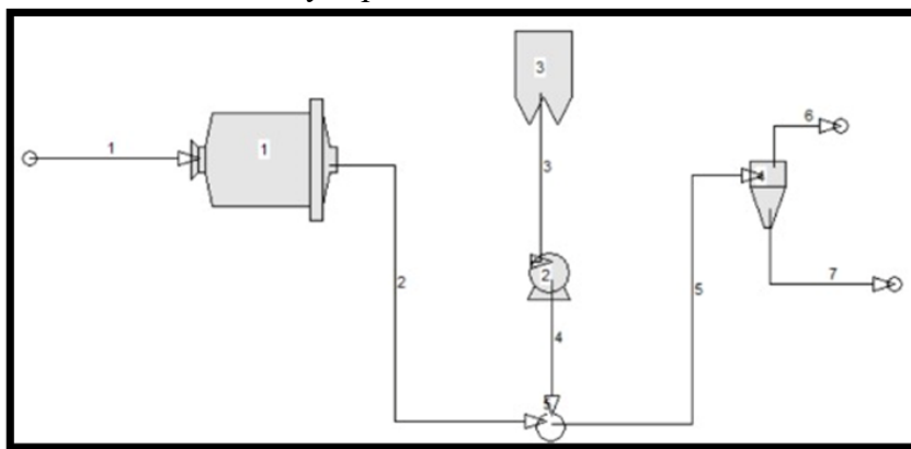
Figura 1. Circuito de molienda y separación con hidrociclón
