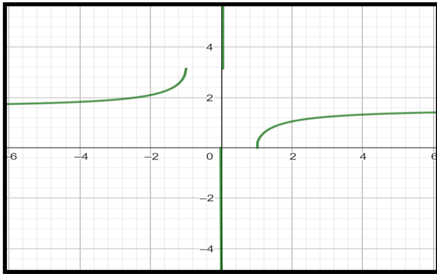
Figura. 3.37 Gráfica de la función \text{arcsec}(x)
