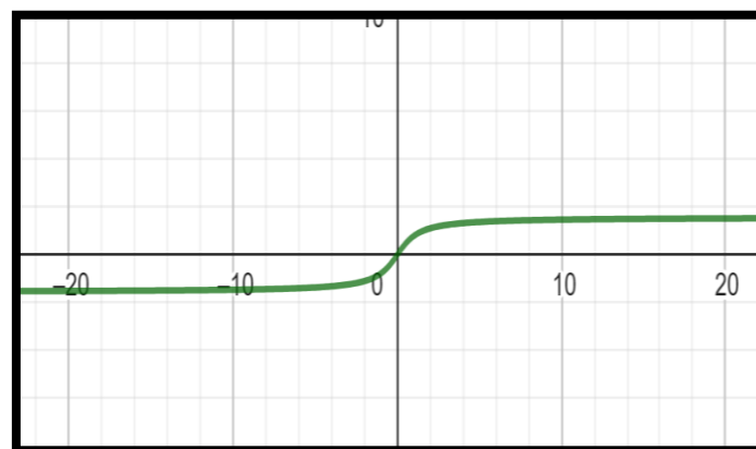
Figura. 3.35 Grafica de la función \arctan(x)
