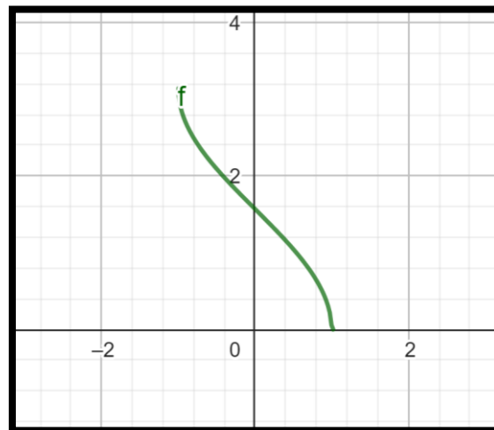
Figura. 3.34 Grafica de la función \arccos(x)
