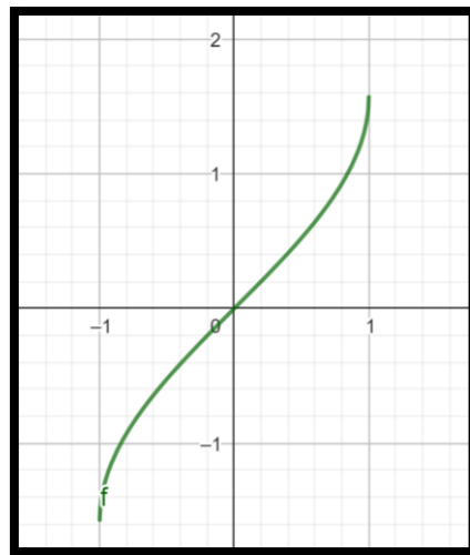
Figura. 3.33 Grafica de la función \text{arcsen}(x)
