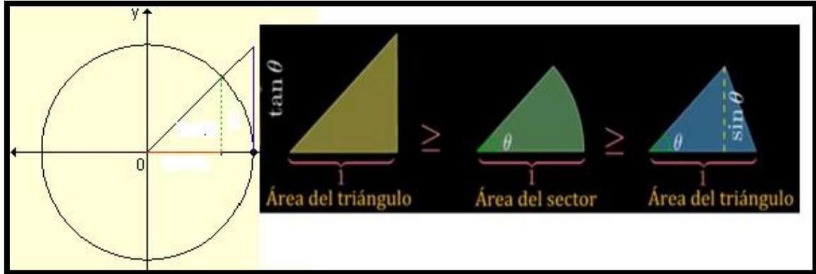
Figura. 2.33 Áreas y ángulos de una circunferencia
