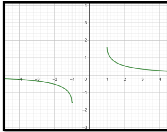
Figura. 3.38 Gráfica de la función \text{arccsc}(x)
